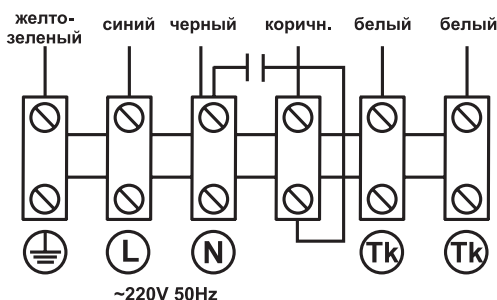
Схема подключения №5
